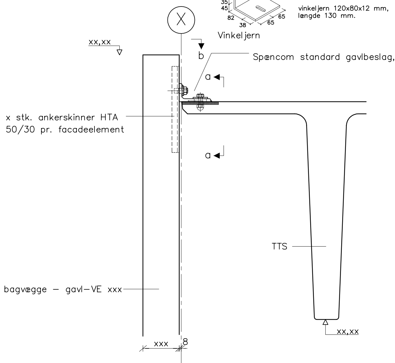
Samling mellem TTS/VE ved gavl med Spæncom standard gavlbleslag
